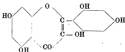
Morin.
